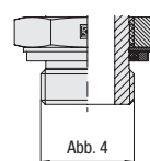
O-Ring mit Kammerring (einstellbar)
