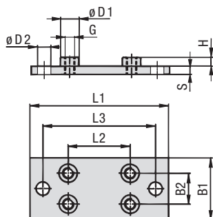
STAUFF Größe 3S bis 9S
