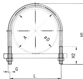
Rundstahlbügel (Typ RBD)
