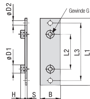
STAUFF Größe 1A bis 8 (7M / 8M)
